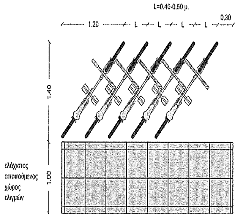
Σχήμα 2: διάταξη θέσεων υπό γωνία σε σειρά
