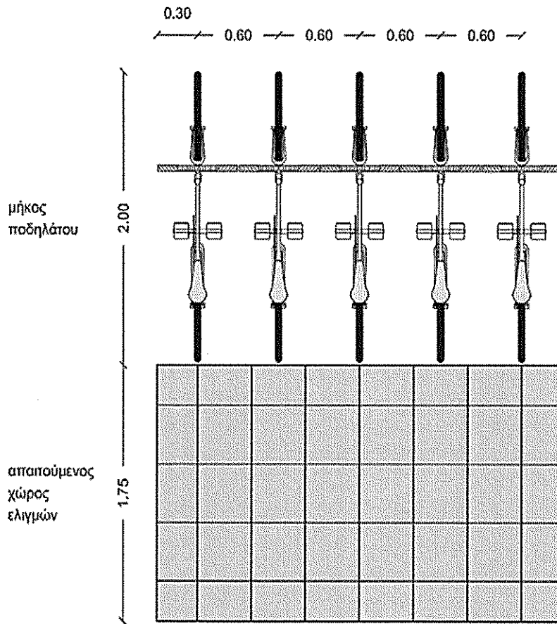
Σχήμα 1: διάταξη θέσεων σε σειρά
