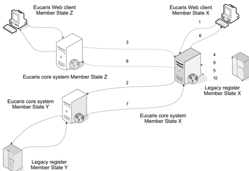
Σχήμα 5: Τύποι μηνυμάτων για καταγραφή
