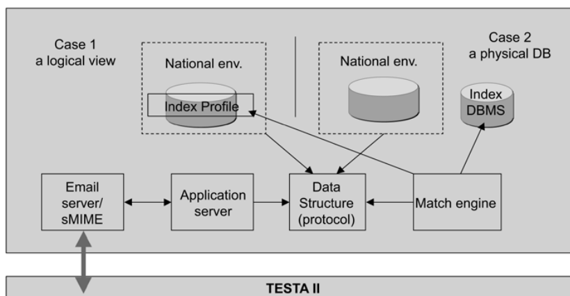
Σχήμα 2: Γενική τοπολογία της εφαρμογής
