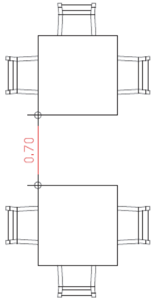
Παράρτημα 4: Παραδείγματα διάταξης τραπεζοκαθισμάτων όπου στον ενδίδμεσο χώρο δεν τοποθετείται κάθισμα.
